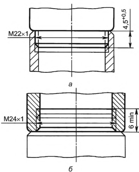
Рисунок 24 — Основные размеры седла клапана и резьб для присоединения вентильных головок
