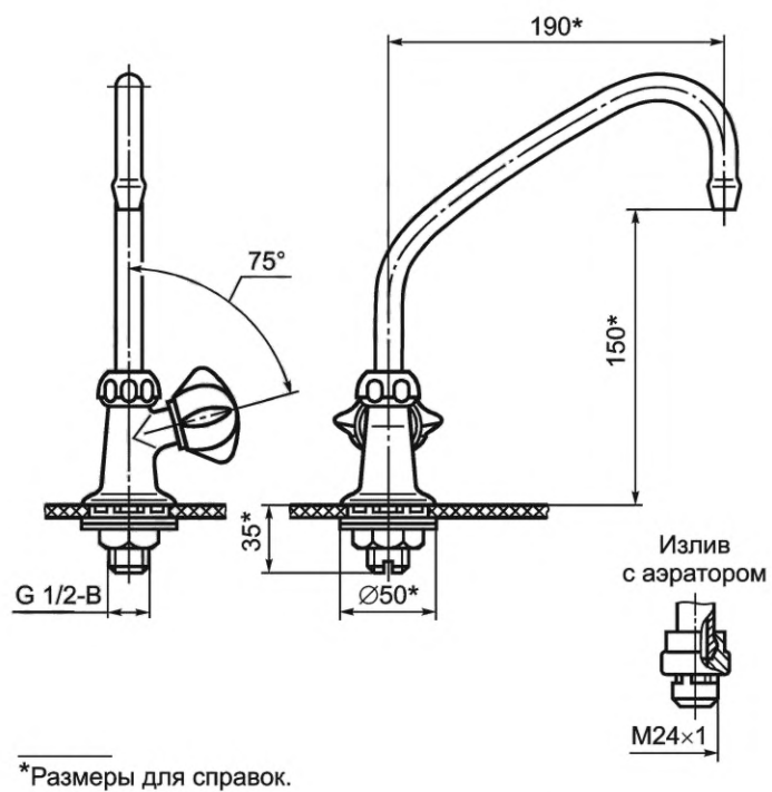
Рисунок 28 — Кран водоразборный напорный (типы КрЦБр, КрЦБА)
