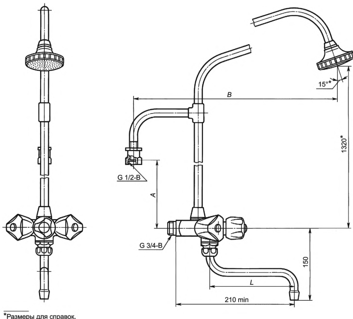
Рисунок 20 — Смеситель для водогрейной колонки двухрукояточный настенный с душевой сеткой на стационарной трубке. Тип См-КДНТр
