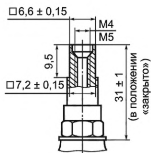
Рисунок 26 — Размеры конца шпинделя вентильных головок водоразборной санитарно-технической арматуры
