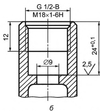
Рисунок 24 — Основные размеры седла клапана и резьб для присоединения вентильных головок
