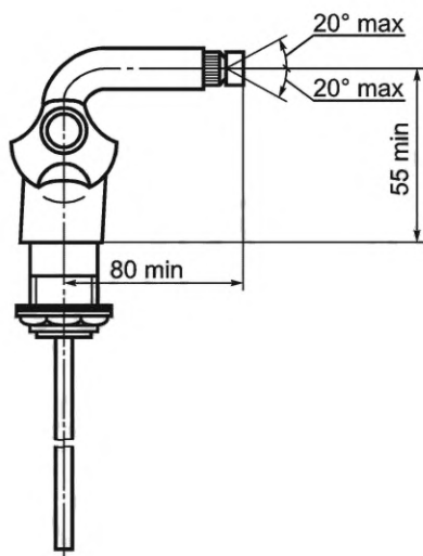
Рисунок 21 — Смеситель для бидэ двухрукоятный центральный набоортный. Тип См-БДДЦБ
