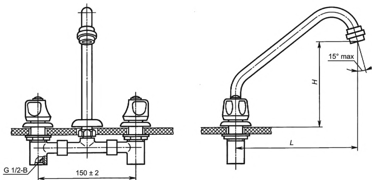
Рисунок 6 — Смеситель для умывальника и мойки двухрукояточный с подводками в раздельных отверстиях набоортный, излив с аэратором. Типы См-УмДРБА, См-МДРБА
