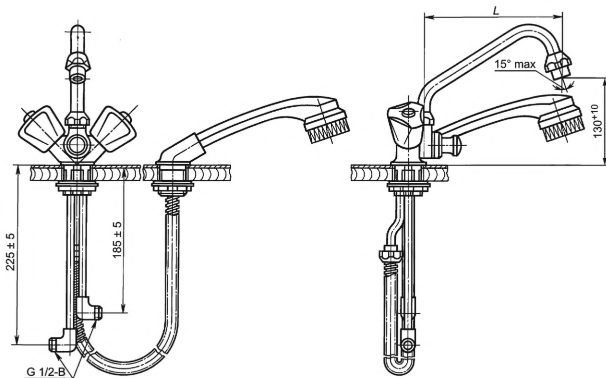
Рисунок 8 — Смеситель для мойки двухрукояточный центральный набо́ртный со щеткой с набо́ртным креплени́ем, излив с аэра́тором. Тип См-МДЦБЩБА
