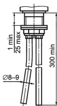
Рисунок 22 — Основные размеры гибких медных подводок для присоединения центральных набоортных смесителей к сетям холодной и горячей воды
